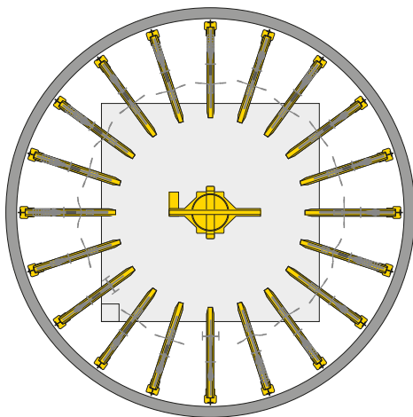
Schnitt Parkebene
