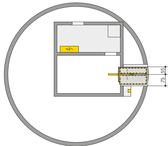
Schnitt Einfahrtsebene
