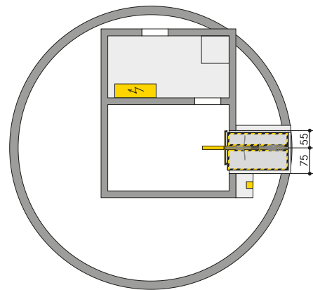
Schnitt Einfahrtsebene
