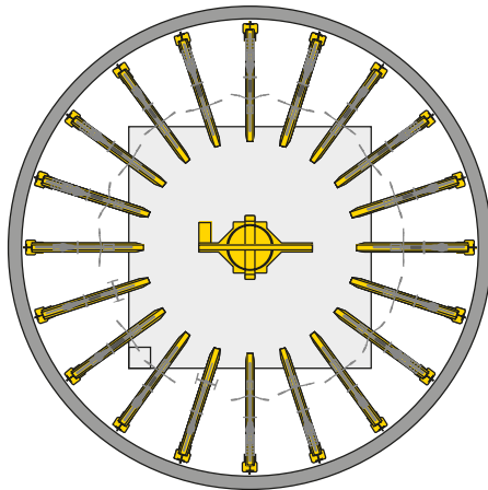
Schnitt Parkebene
