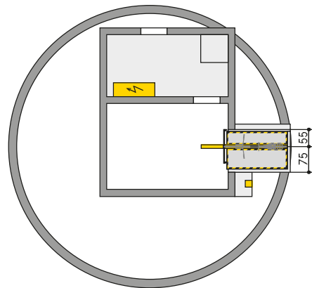
Schnitt Einfahrtsebene
