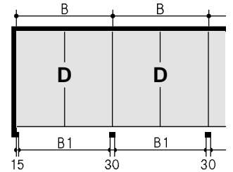
Reihengarage mit Doppeltoren (je 4 Pkw)
