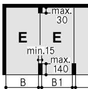
Einzelanlage (2 Pkw)
