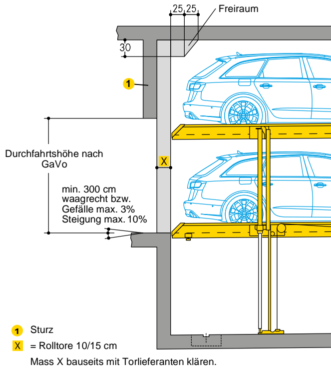
Einzelanlage (2 Pkw)
