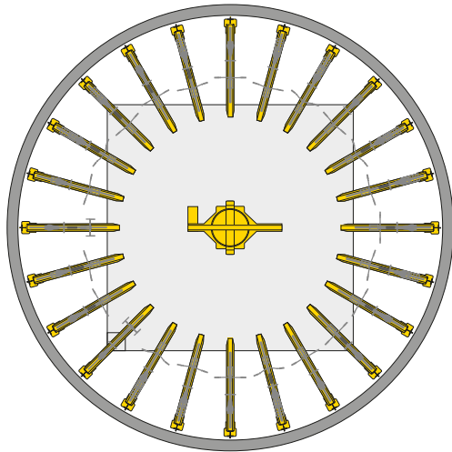
Schnitt Parkebene
