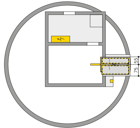
Schnitt Einfahrtsebene
