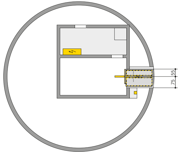
Schnitt Einfahrtsebene
