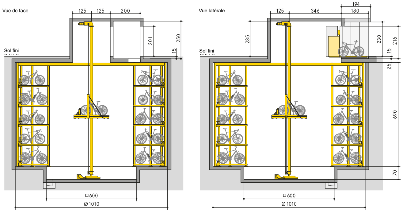
Coupe niveau de parking
