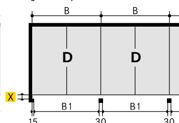
Reihengarage mit Doppeltoren (je 4 Pkw)
