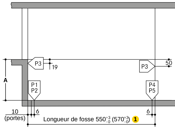
Coupe
